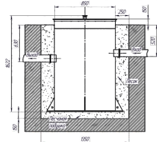
Схема монтажа Малахит AIR 2
