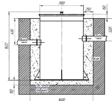
Схема монтажа Малахит AIR 4
