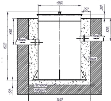
Схема монтажа Малахит AIR 3
